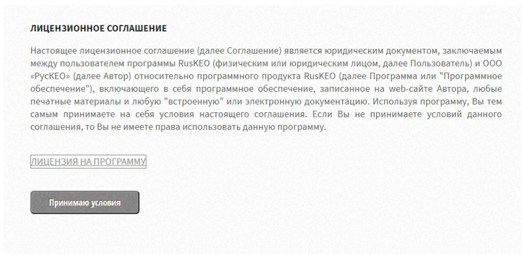
Рисунок 4.2: Лицензионное соглашение
