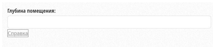
Рисунок 1.1: Справка
