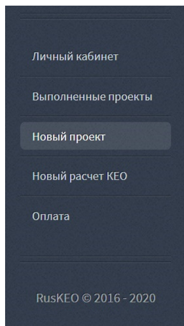
Рисунок 4.1: Новый проект
