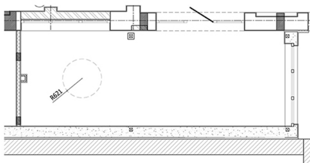
Рисунок 13.7 – Определение радиуса светового фонаря
