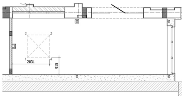
Рисунок 13.13 – Определение координат «Х» и «Y» второй вершины (правой нижней) квадратного/прямоугольного светового фонаря
