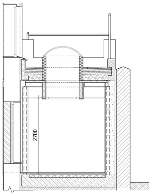
Рисунок 11.4 – Пример определения высоты помещения
