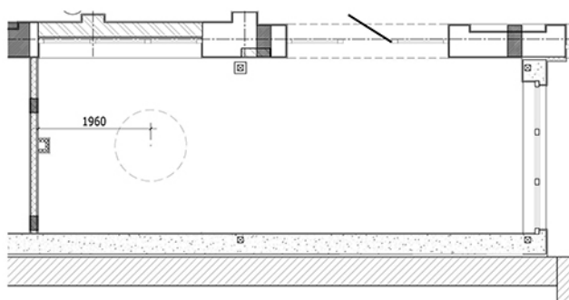
Рисунок 13.5 – Определение координаты «X» центра фонаря относительно нижнего левого угла помещения
