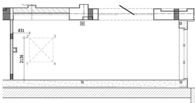
Рисунок 13.12 – Определение координат «X» и «Y» первой (левой верхней) вершины квадратного/прямоугольного светового фонаря
