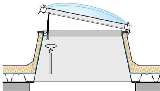
Рисунок 12.5 – Зенитный фонарь
